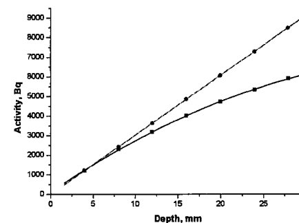
Рис. 2.5. Измеренная интегральная наведенная активность в зависимости от толщины мишени (■ точки), и вычисленные значения наведенной активности в предположении, что во всех таблетках наведенная активность одинакова (● точки).
