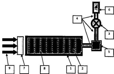
Рис. 1.5. Схема газовой мишени
