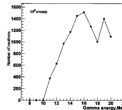
Рис. 3.1. Зависимость выхода нейтронов от энергии фотонов при облучении ксенона.
