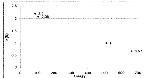
Рис. 1.6. Зависимость эффективности (в процентах) регистрации гамма-квантов детектором \text{NaI}(\text{Tl}) от энергии на расстоянии 10 см от входного окна.
