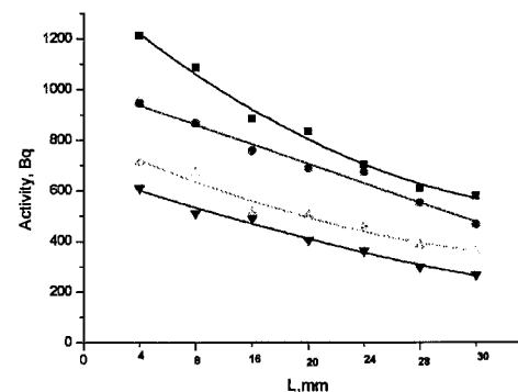
Рис. 2.4. Зависимость измеренной активности облученной мишени \text{MoO}_3 от глубины через ■ – 15.7 часа, ● - 37.8 часа, ▲- 62.7 час и ▼- 84.3 часа после завершения облучения
