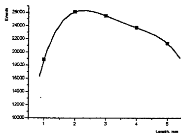
Рис. 1.1 Зависимость выхода фотонов от толщины танталового радиатора.
