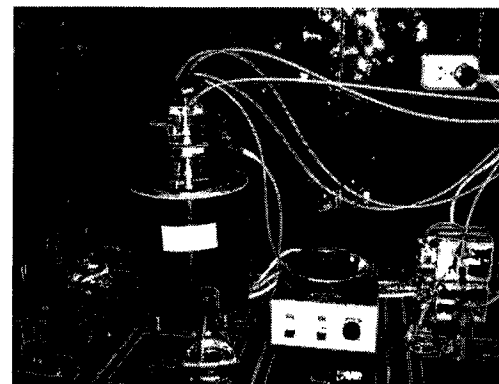
Рис. 2.7. Экстрактор, мешалка и перистальтические насосы в вытяжном шкафу.
