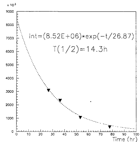
Рис. 3.3. Зависимость активности выделенного изотопа ^{123}\text{I} от времени после завершения облучения.
