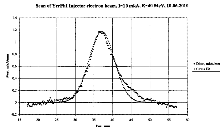
Рис. 1.3. Результат измерения профиля пучка в вертикальном направлении.
