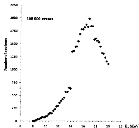
Рис. 2.1. Зависимость числа нейтронов, вылетевших из мишени ^{100}\text{Mo} толщиной 1 см от энергии фотонов (каждая точка является результатом от 10^5 фотонов).
