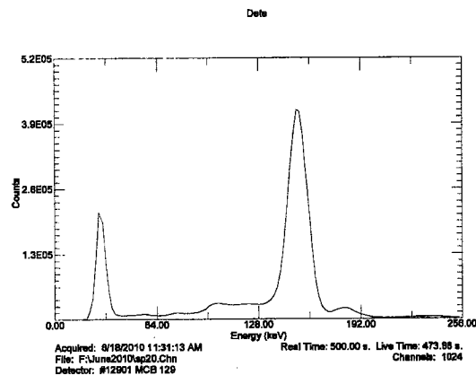
Рис.3.2. Спектр излучения выделенного ^{123}\text{I} через 26 часов после завершения облучения.
