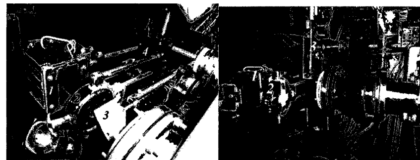
Рис. 1.2. Экспериментальная установка под электронным пучком. 1 - цилиндр Фарадея, 2 – мишенный модуль, 3-люминифорный экран контроля позиции пучка, 4 – дистанционное устройство передвижения мишенного модуля.
