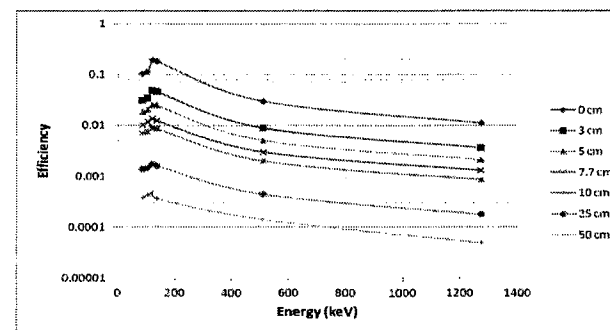
Рис. 1.7. Эффективность детектора из сверхчистого германия на расстояниях 0, 3, 5, 7.7, 10, 25 и 50 см от источника до детектора.
