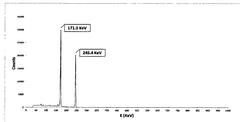
Рис. 4.1. Гамма-спектр облученного материала через 332 часа после экспозиции.
